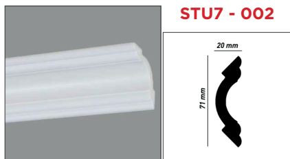
2000 x 20 x 71 mm / Kunststoff
