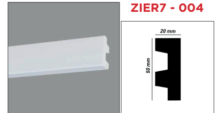
2000 x 20 x 50 mm / Kunststoff
