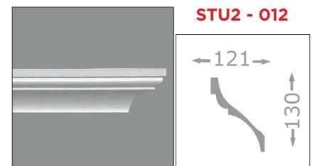
2000 x 121 x 130 mm / Polystyrol
